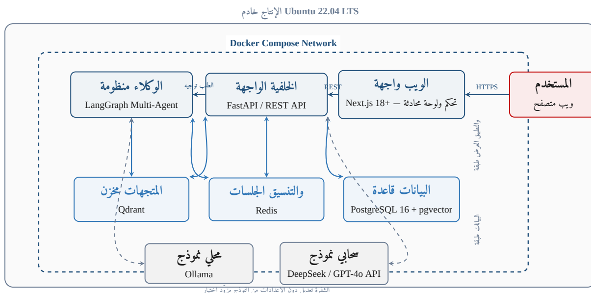
شكل 3-4: معمارية نشر نظام «بيان» عبر Docker Compose.
