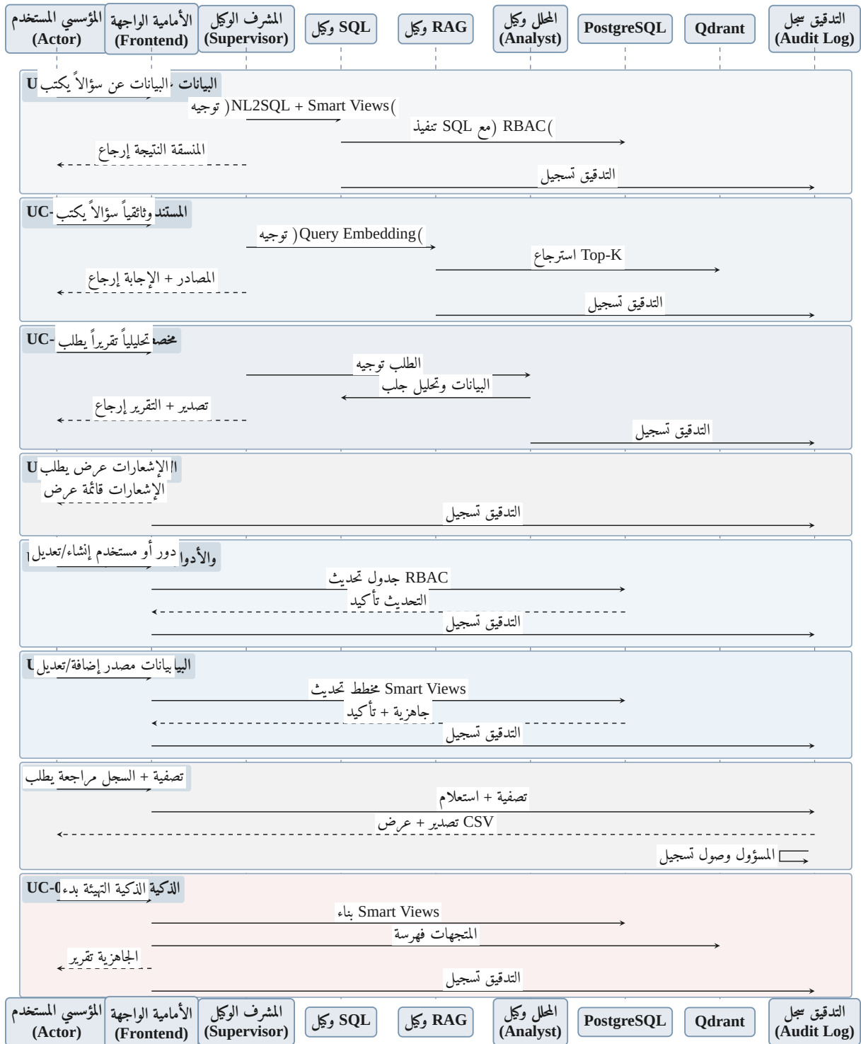
شكل 3-7: مخطط التسلسل الشامل لحالات الاستخدام الثماني (UC-01) إلى (UC-08) في نظام «بيان»، يُظهر التدفق الزمني للرسائل بين المكونات التسعة الرئيسية.
