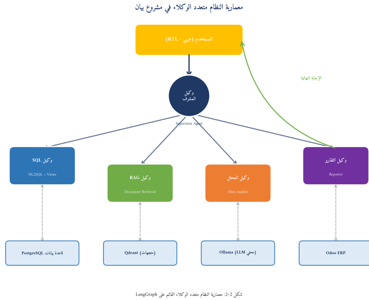
شكل 2.2: معمارة النظام متعدد الوكلاء القائم على LangGraph.
