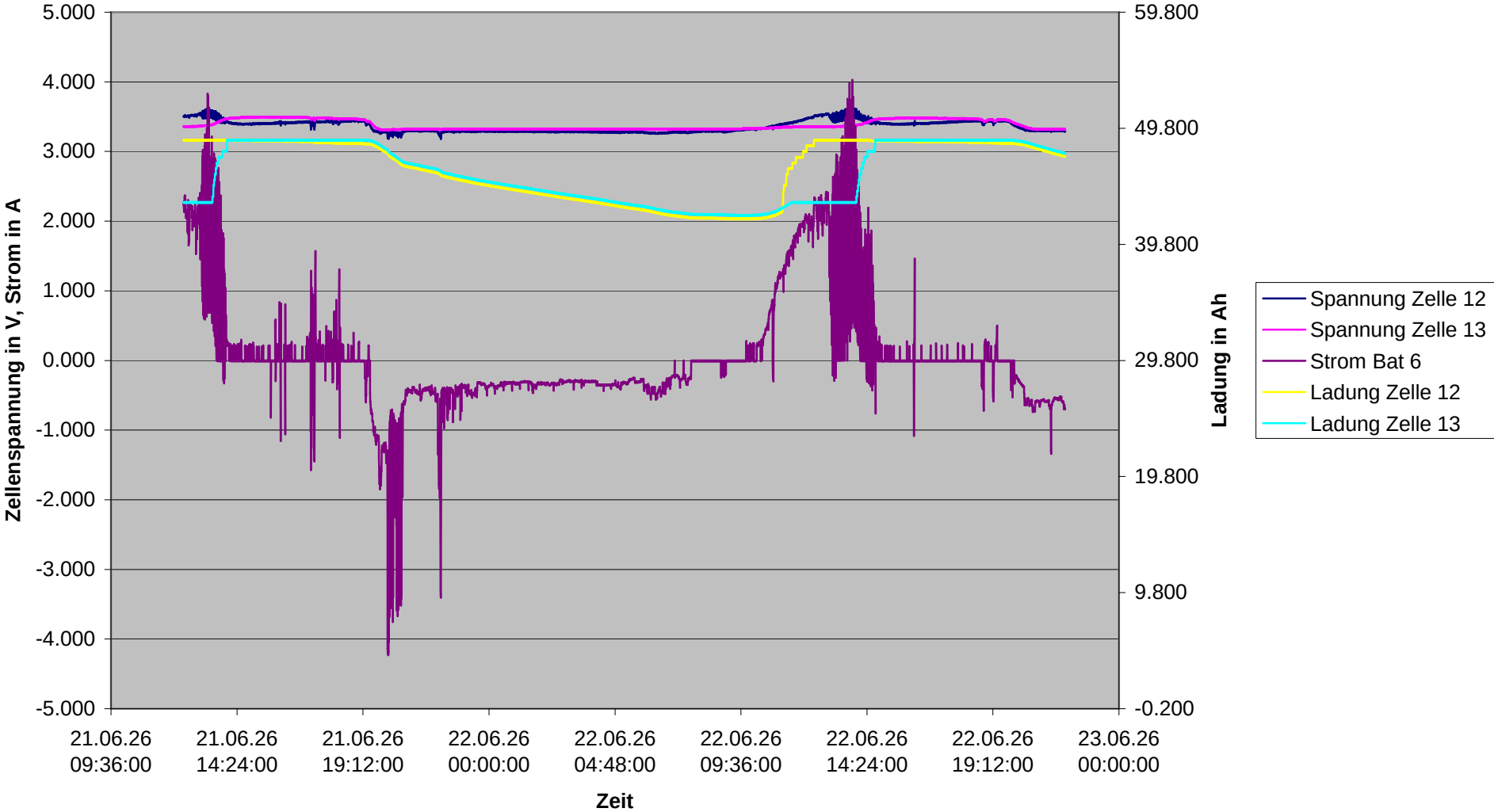
Batterie 6, Zelle 12 im Vergleich zu Zelle 13
