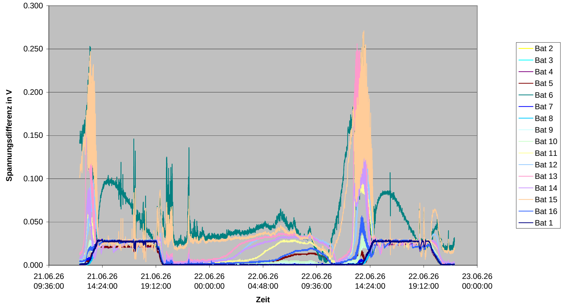
Spannungsdifferenz (höchste Zellspannung - niedrigste Zellspannung)
