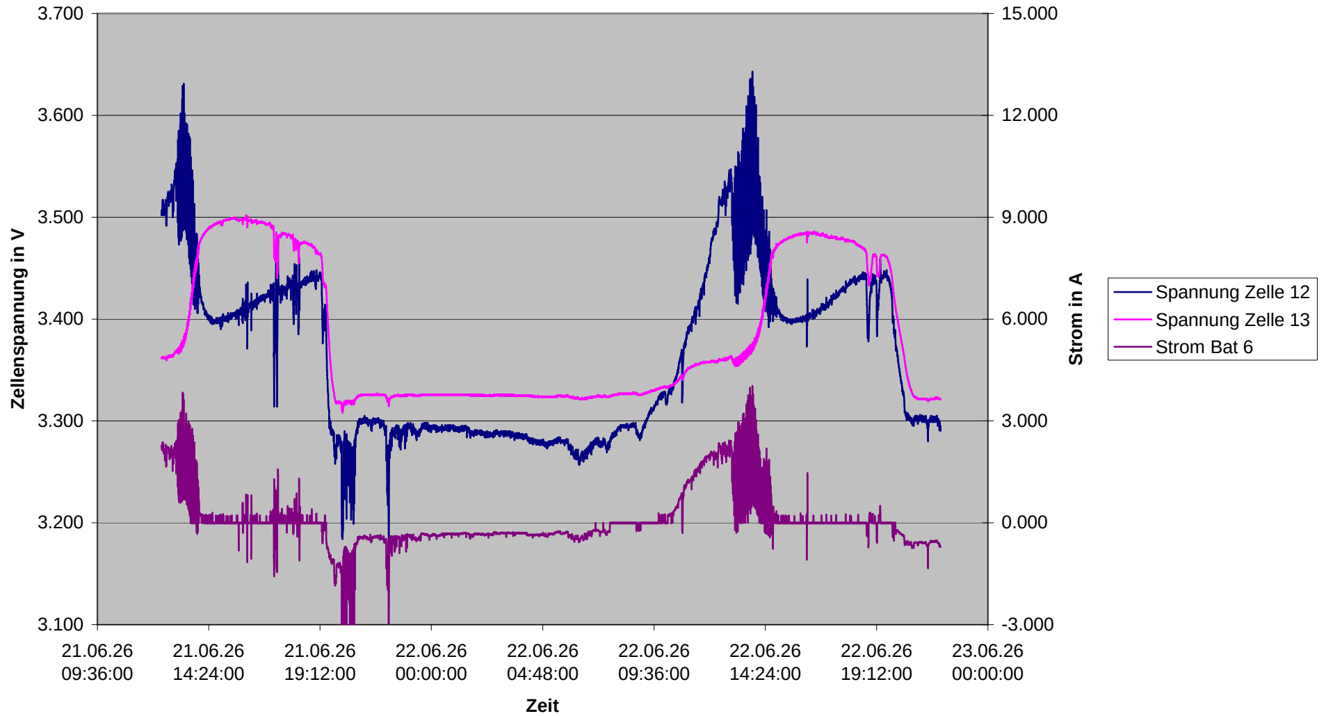
Spannung und Strom bei Batterie 6, Zelle 12 im Vergleich zu Zelle 13
