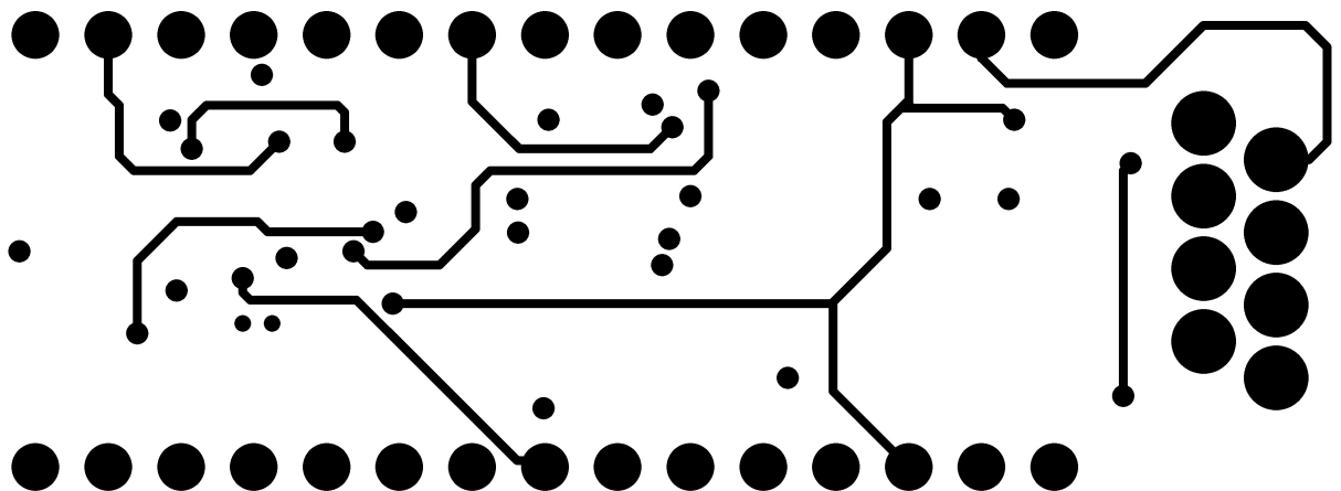
Copper Layer 15
