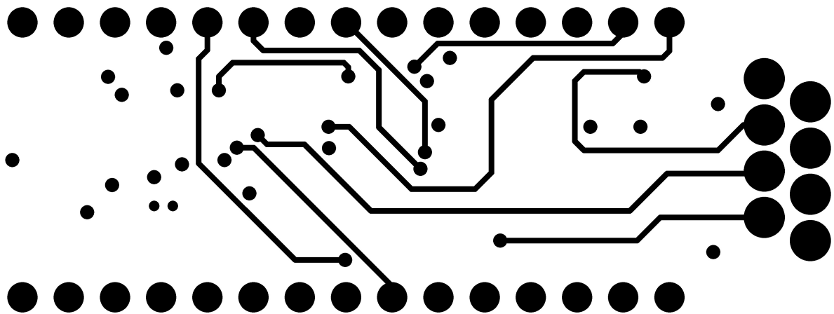
Copper Layer 2
