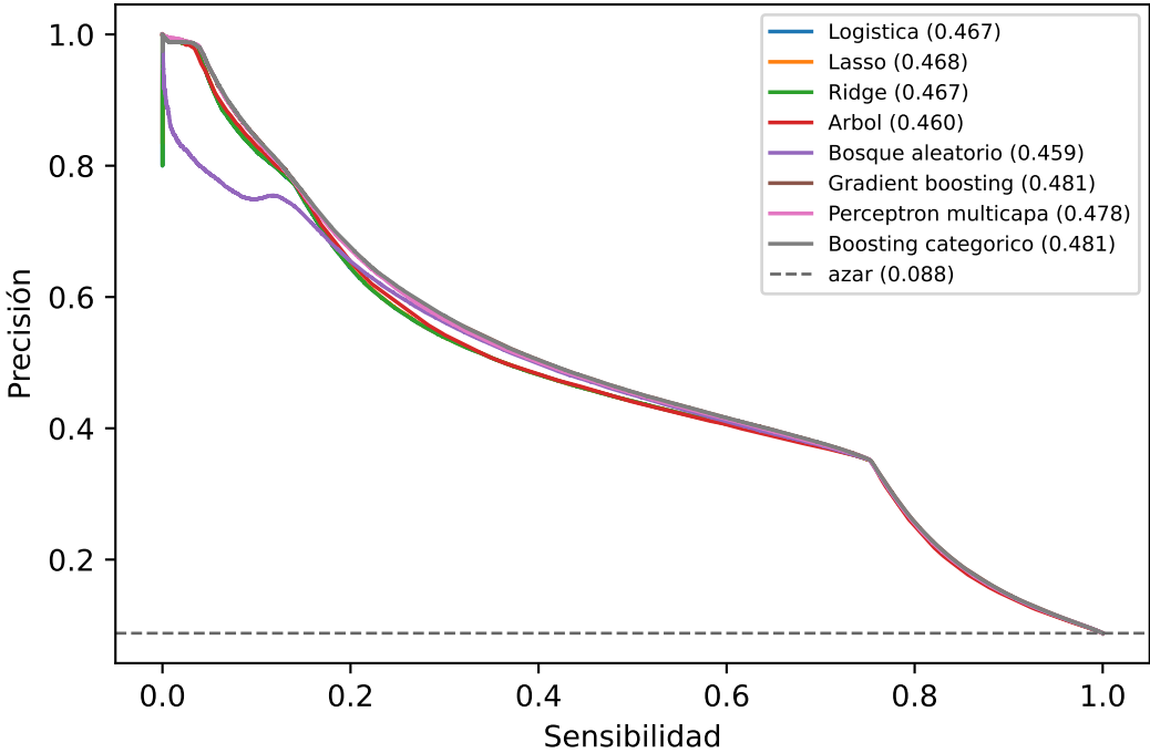
(a) Precisión-sensibilidad
