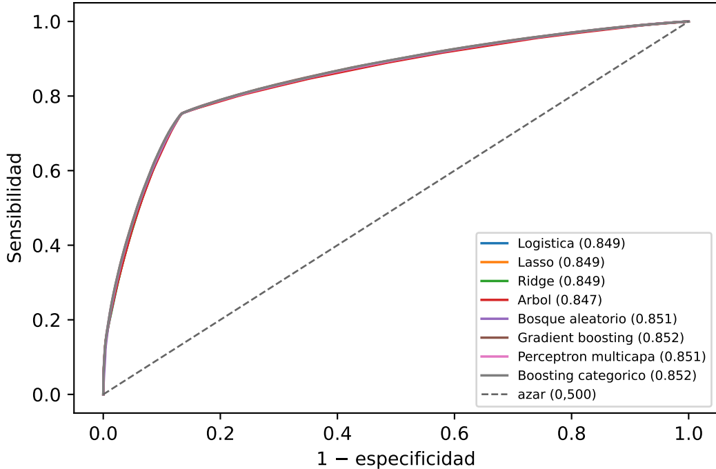
(b) ROC
