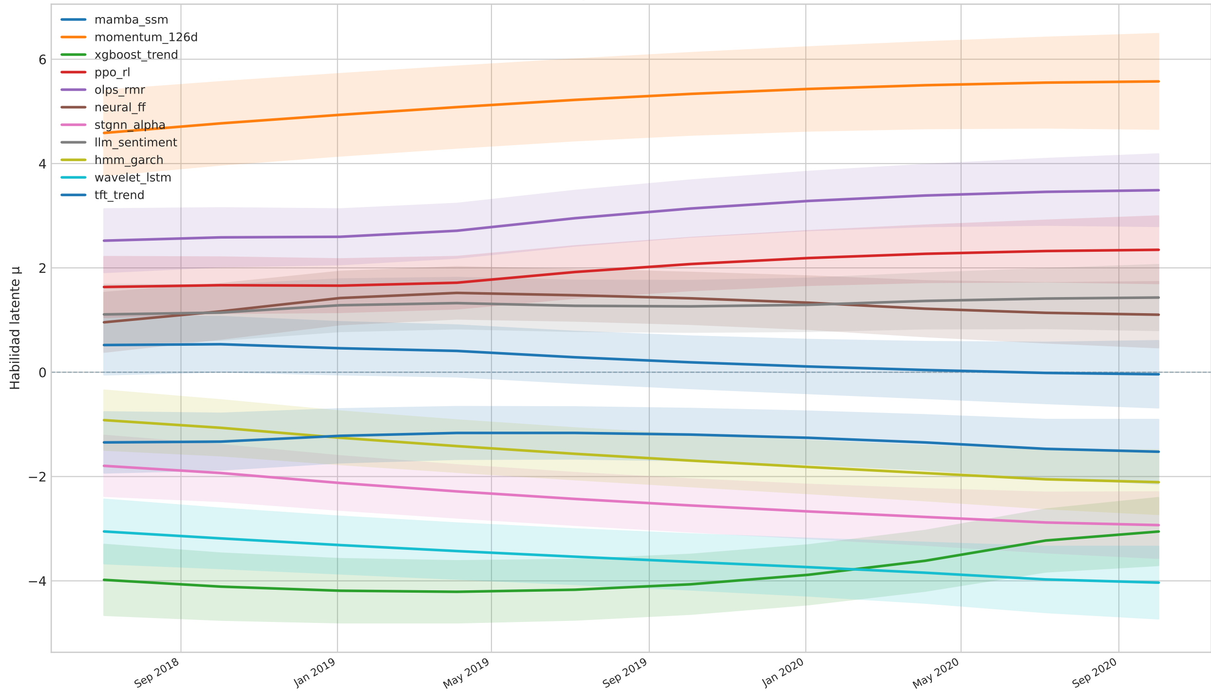
Curvas de Aprendizaje TTT — \mu \pm 1\sigma por Estrategia
