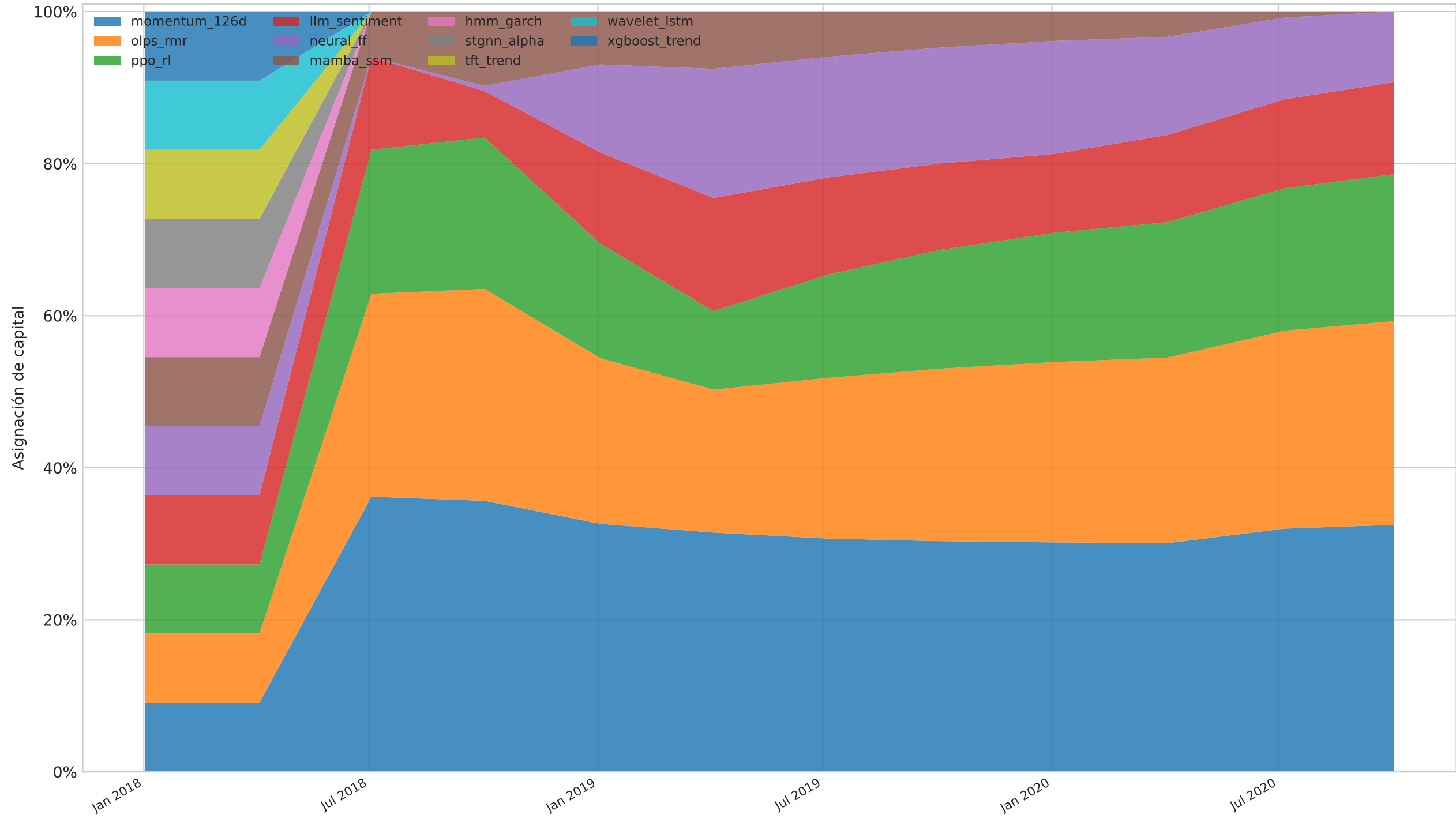
Asignación Dinámica del Juez TTT por Estrategia
