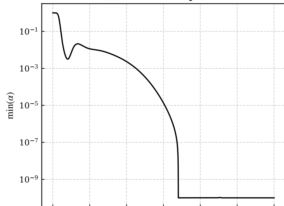
(d) Max trapped surface radius: \theta_+ \leq 0
