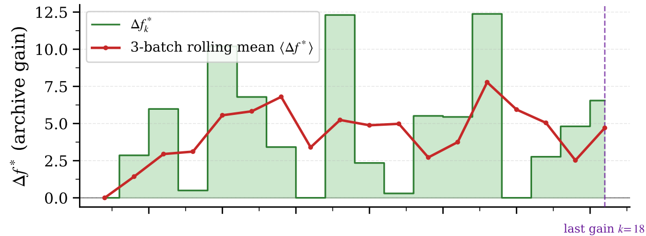
CMA-ES refinement progress — ftl_4d_cmaes_v1
