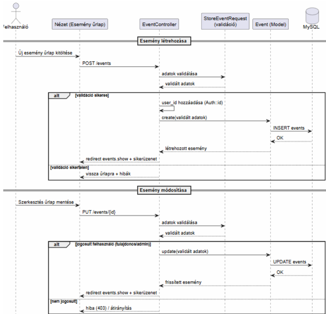
9.1. ábra: Az esemény létrehozásának és módosításának szekvenciadiagramja
