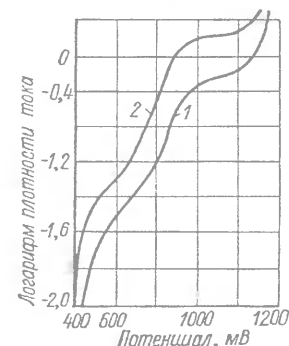
Рис. 7. Поляризационные кривые золота (г/л) в щелочном цианистом электролите:
