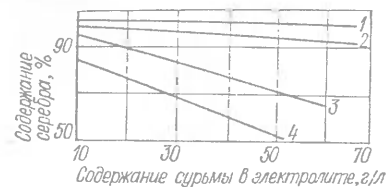
Рис. 4. Зависимость состава покрытия от содержания сурьмы в электролите и плотности тока (А/дм 2 ):
