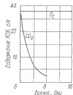
Рис. 2. Зависимость содержания цианистого калия в ванне серебрения от времени пропускания кислорода и углекислого газа
