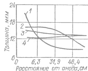
Рис. 6. Распределение золота на различных удаленных от анода катодах:
