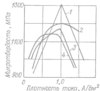
Рис. 5. Влияние плотности тока и различного содержания никеля (г/д) в цианистом электролите на микротвердость серебра: 1 — 0,5; 2 — 1,0; 3 — 2,0; 4 — 7,0
