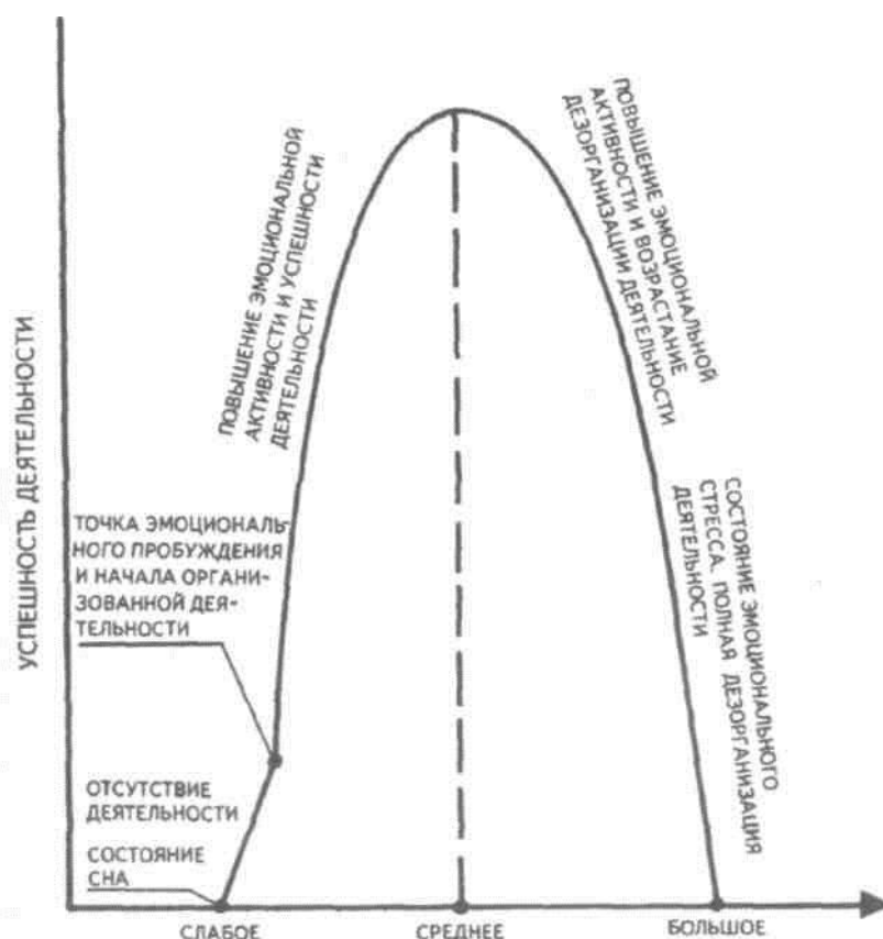
Рис. 3. Зависимость успешности деятельности человека от силы его эмоционального возбуждения (по Д.О.Хеббу)
