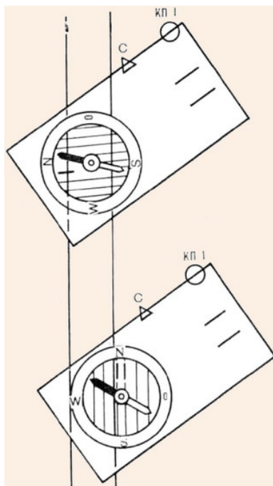
Рис. 3. Установка азимута на спортивном компасе
