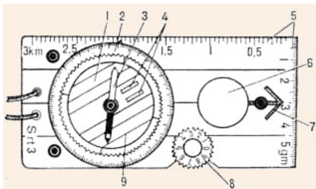
Рис. 1. Спортивный (жидкостный) компас
