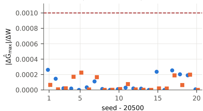
|\hat{G}_{\max} \text{ dev} - \text{final}| (G-N)
