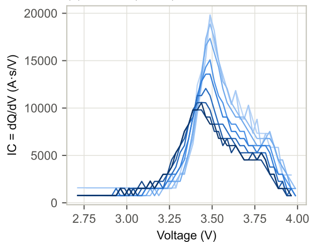
(d) IC curve ( dQ/dV )
