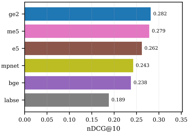
IT-RAG-Bench nDCG@10
