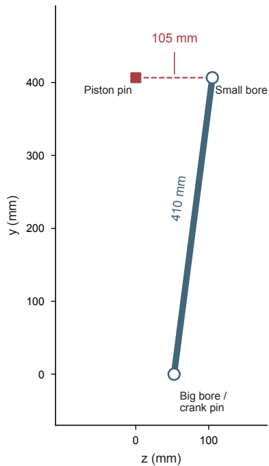
a Actual rod centres at 90°
