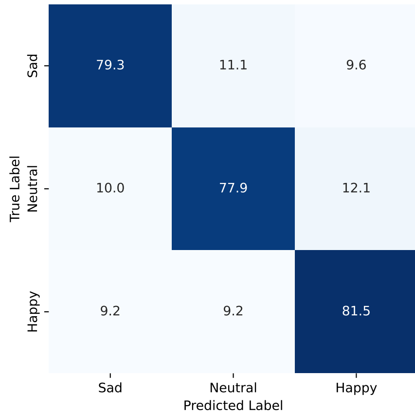
(d) DBN
