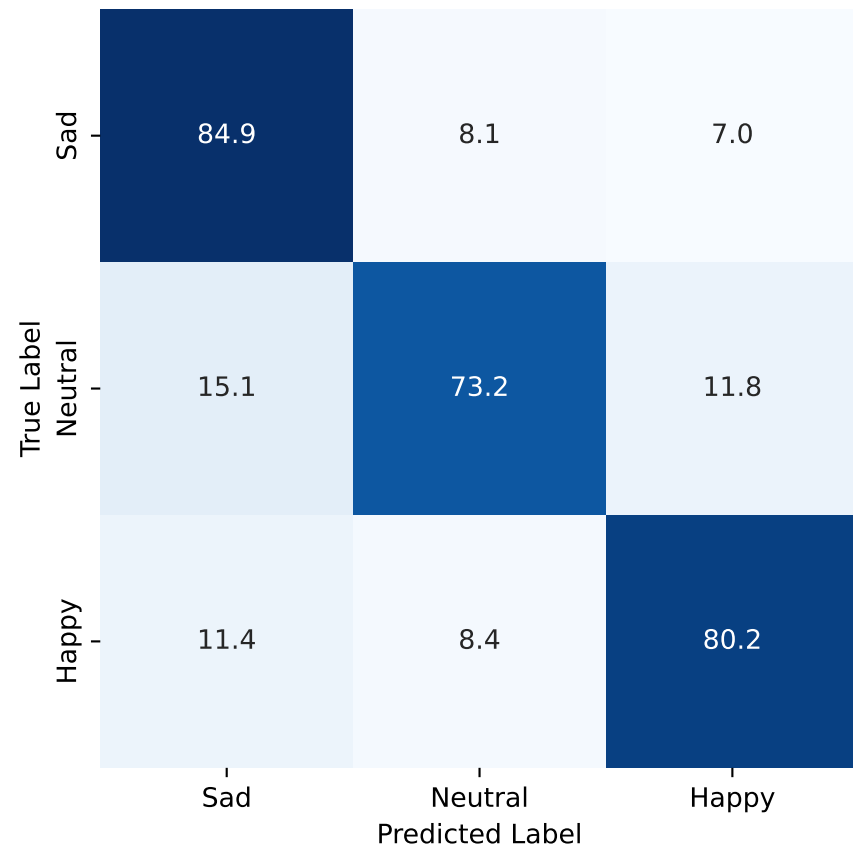
(d) DBN
