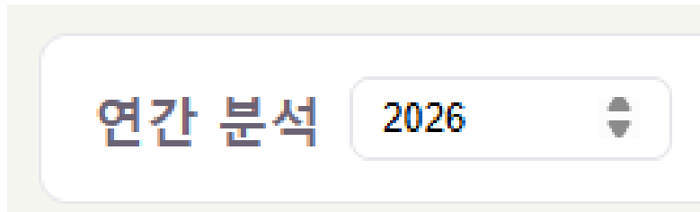
그림 6-1 연도 입력
