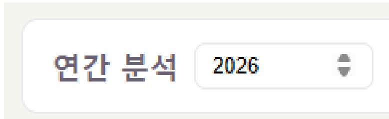
그림 6-1 연도 입력
