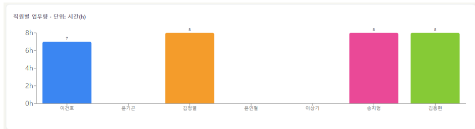
그림 7-1 직원별 업무량
