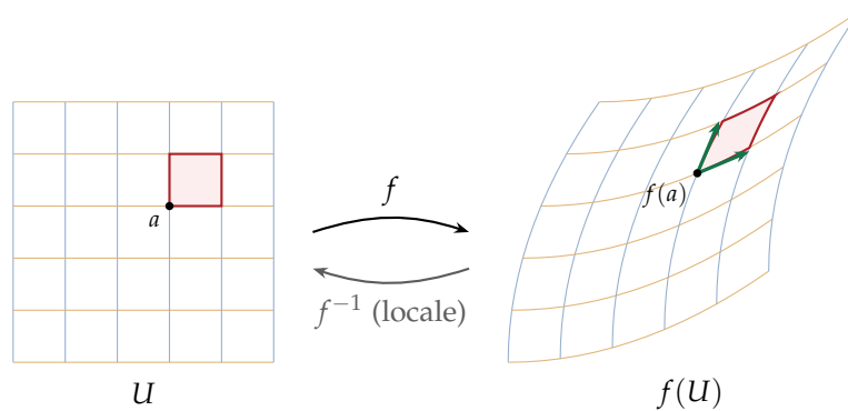
Figure 3.1. Inversion locale pour f(x, y) = (x + 0,35y^2, y + 0,35x^2) . Un petit carreau issu de a est envoyé sur un quadrilatère curviligne très proche du parallélogramme construit sur les images par df_a des côtés (flèches vertes). Si ce parallélogramme n'est pas aplati ( \det \text{Jac}_f(a) \neq 0 ), f est bijective au voisinage de a .
