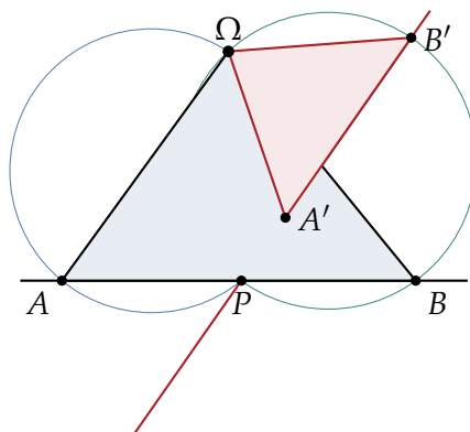
Figure 3.7. Centre \Omega de la similitude directe envoyant A, B sur A', B' (ici de rapport 0,62 et d'angle 55^\circ ) : c'est le second point commun des cercles (PAA') et (PBB') , où P = (AB) \cap (A'B') . Les triangles \Omega AB et \Omega A'B' sont directement semblables.
