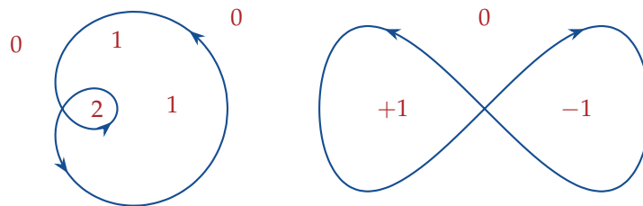
Figure 3.2. Indices de deux lacets, constants sur chaque composante connexe du complémentaire. À gauche, un limaçon (de Pascal) parcouru dans le sens direct : indice 2 dans la petite boucle, 1 entre les deux boucles, 0 dehors. À droite, une lemniscate : les deux lobes sont parcourus en sens contraires, d'indices -1 et +1 .
