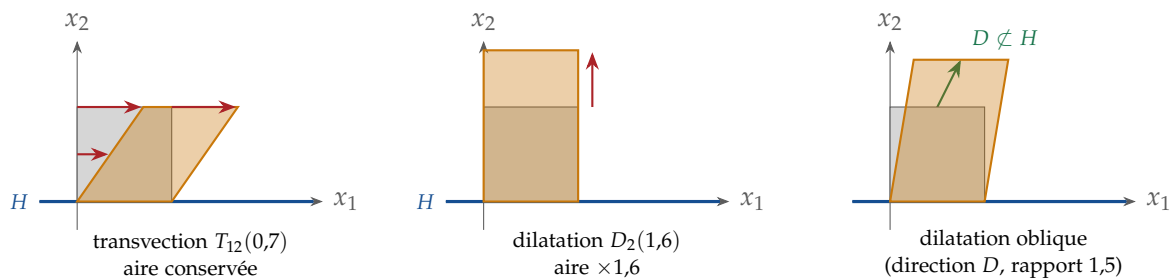
Figure 2.1. Image du carré unité. Les trois applications fixent l'hyperplan H (l'axe x_1 ) point par point. La transvection fait glisser les points parallèlement à H , proportionnellement à leur hauteur : l'aire est conservée. Une dilatation déplace les points selon une direction D hors de H et multiplie l'aire par son rapport \det u .
