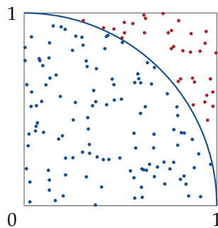
Figure 7.3. Monte-Carlo pour \frac{\pi}{4} = \mathbb{P}(U_1^2 + U_2^2 \leq 1) : 150 points uniformes dans le carré, dont 116 dans le quart de disque (bleu), d'où l'estimation 4 \times \frac{116}{150} \approx 3,09 .
