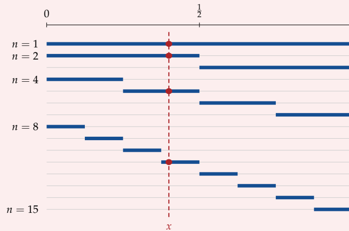
Figure 5.3. La machine à écrire : le support de f_n (en bleu) balaie indéfiniment [0, 1] en rétrécissant. Chaque point x est visité une fois par ligne dyadique, donc une infinité de fois.
