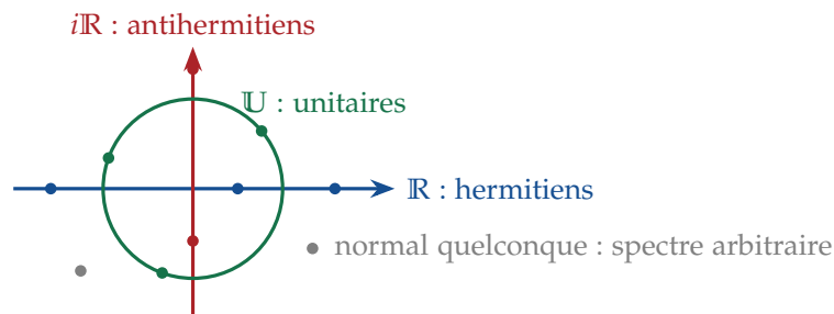
Figure 7.1. Les endomorphismes normaux sont diagonalisables en base orthonormée ; les trois familles classiques se distinguent par la position de leur spectre.
