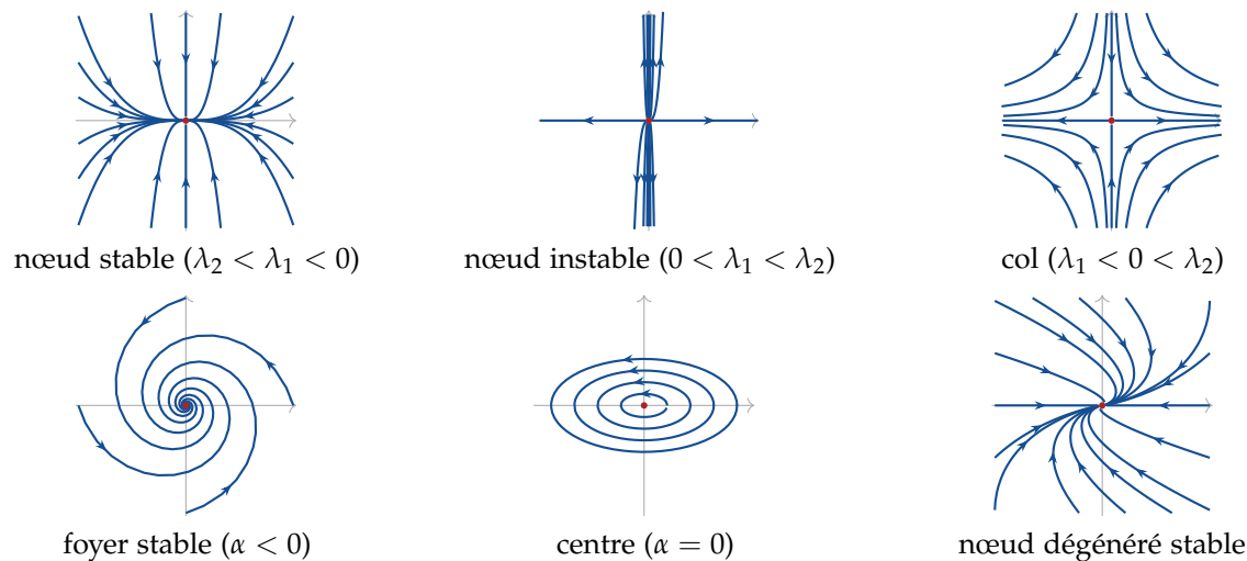
Figure 8.1. Les six portraits de phase génériques de y' = Ay dans le plan (trajectoires calculées exactement par e^{tA} ). Les nœuds instables sont les nœuds stables parcourus en sens inverse; de même pour les foyers.
