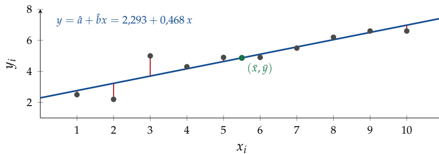
Figure 8.2. Régression linéaire simple de l'exemple 8.3 : droite des moindres carrés (bleu), qui passe par le point moyen (\bar{x}, \bar{y}) , et résidus \hat{\epsilon}_i = y_i - \hat{a} - \hat{b}x_i (segments rouges). La méthode minimise la somme des carrés des longueurs verticales des segments.
