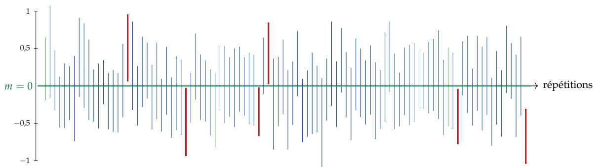
Figure 5.1. Cent intervalles de Student de niveau 95 %, simulés pour n = 20 observations \mathcal{N}(0, 1) (graine fixée). Chaque répétition donne un intervalle différent ; ici 6 sur 100 manquent la vraie valeur m = 0 (en rouge), en accord avec la fréquence théorique 5 %. La probabilité porte sur l'intervalle, pas sur m .
