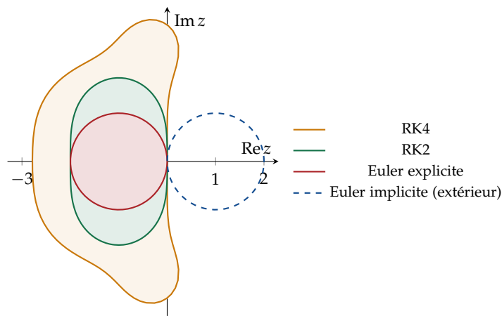
Figure 8.2. Régions de stabilité absolue \{|R(z)| < 1\} : intérieur du disque D(-1, 1) pour Euler explicite, des courbes verte et orange pour RK2 et RK4 (elles coupent l'axe réel en -2 et -2,79 ), extérieur du disque D(1, 1) pour Euler implicite. Les régions des schémas explicites sont bornées.
