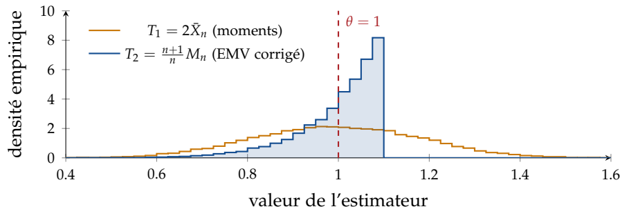
Figure 1.2. Histogrammes de 20 000 réalisations simulées de T_1 et T_2 pour n = 10 , \theta = 1 (graine fixée). Les deux sont centrés en \theta , mais T_2 est quatre fois plus concentré (variances empiriques 0,0335 et 0,0086, contre \frac{1}{30} et \frac{1}{120} en théorie). Sa loi, à support [0, \frac{n+1}{n}\theta] , est très dissymétrique.
