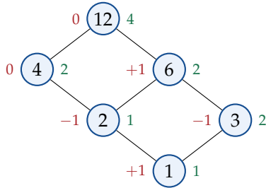
Figure 8.1. Inversion de Möbius sur le treillis des diviseurs de 12 : \varphi * \mathbf{1} = \text{id} (formule de Gauss) s'inverse en \varphi = \mu * \text{id} .
