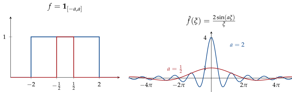
Figure 7.1. Porte et sinus cardinal, pour a = 2 (bleu) et a = \frac{1}{2} (rouge) : une porte large a une transformée haute, étroite et très oscillante ; une porte étroite a une transformée basse et étalée. La décroissance n'est qu'en \frac{1}{|\xi|} .
