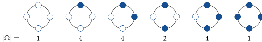
Figure 1.3. Les 6 colliers à 4 perles et 2 couleurs : un représentant par orbite de \mathbb{Z}/4\mathbb{Z} agissant sur les 16 coloriages. Sous chaque collier, le cardinal de l'orbite ; on vérifie 1 + 4 + 4 + 2 + 4 + 1 = 16 .
