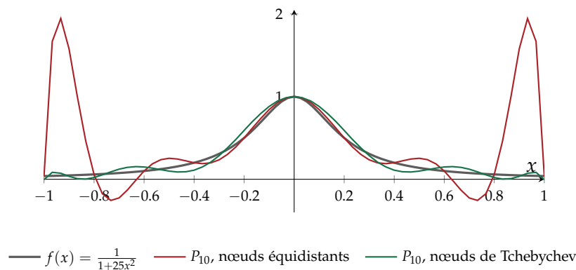
Figure 13.2. Phénomène de Runge : avec 11 nœuds équidistants, l'erreur uniforme vaut déjà environ 1,9 et tend vers l'infini avec n ; avec les nœuds de Tchebychev elle vaut environ 0,11 et tend vers 0. Ce n'est pas un défaut de régularité de f (qui est analytique sur \mathbb{R} ) mais de ses pôles \pm \frac{i}{5} et de la répartition des nœuds.
