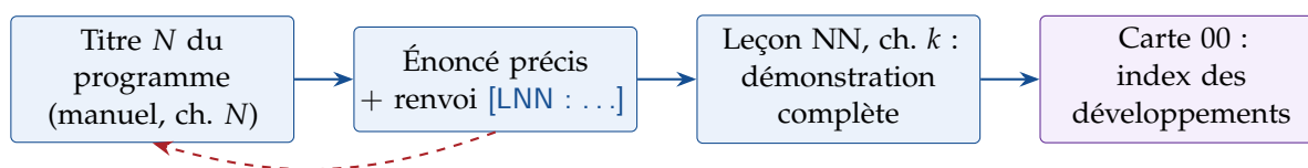
Figure 0.1. Le circuit de lecture : du programme vers l'énoncé, de l'énoncé vers la preuve, de la preuve vers le développement d'oral.
