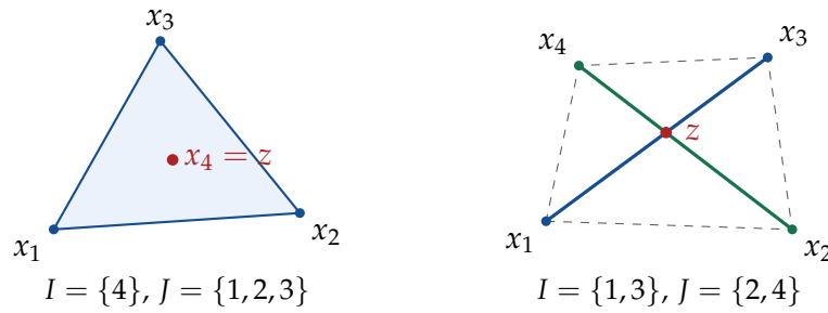
Figure 5.2. Le théorème de Radon dans le plan ( n + 2 = 4 points) : soit un point est dans le triangle des trois autres, soit les quatre points sont en position convexe et les deux diagonales se coupent.
