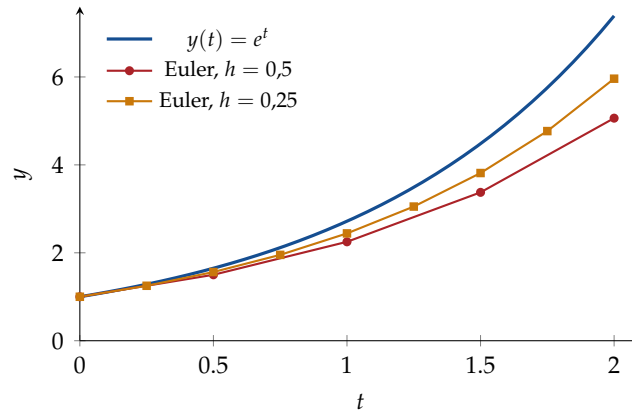
Figure 8.1. Euler explicite pour y' = y , y(0) = 1 : chaque segment suit la pente au point de départ, et la solution approchée reste sous la solution (convexe). En t = 2 , l'erreur vaut 2,33 puis 1,43 : elle est grossièrement divisée par 2 quand h l'est (ordre 1 : asymptotiquement, l'erreur en t est \sim \frac{t e^t}{2} h ).
