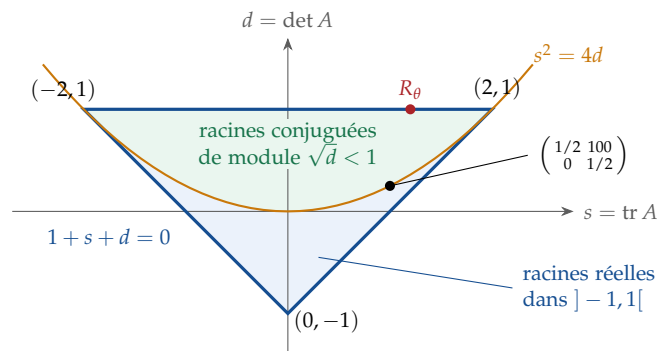
Figure 7.1. Région de stabilité \{\rho(A) < 1\} pour A \in \mathcal{M}_2(\mathbb{R}) , dans le plan (\text{tr } A, \det A) : le triangle ouvert |d| < 1 , |s| < 1 + d (critère de Schur–Cohn). Au-dessus de la parabole s^2 = 4d , valeurs propres complexes conjuguées; en dessous, réelles. Les rotations R_\theta sont sur le côté d = 1 (frontière, \rho = 1 ); la matrice \begin{pmatrix} 1/2 & 100 \\ 0 & 1/2 \end{pmatrix} est sur la parabole, dans la région : ses puissances tendent vers 0 malgré \|A\| \geq 100 . La région ne dépend que de (s, d) , pas de la taille des coefficients : elle est ouverte, non bornée dans \mathcal{M}_2(\mathbb{R}) , et non convexe (exercice 4 du chapitre 9). Critère vérifié numériquement sur 2 \cdot 10^5 tirages.
