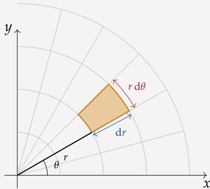
Figure 6.2. Coordonnées polaires : l'élément d'aire vaut r \, dr \, d\theta .
