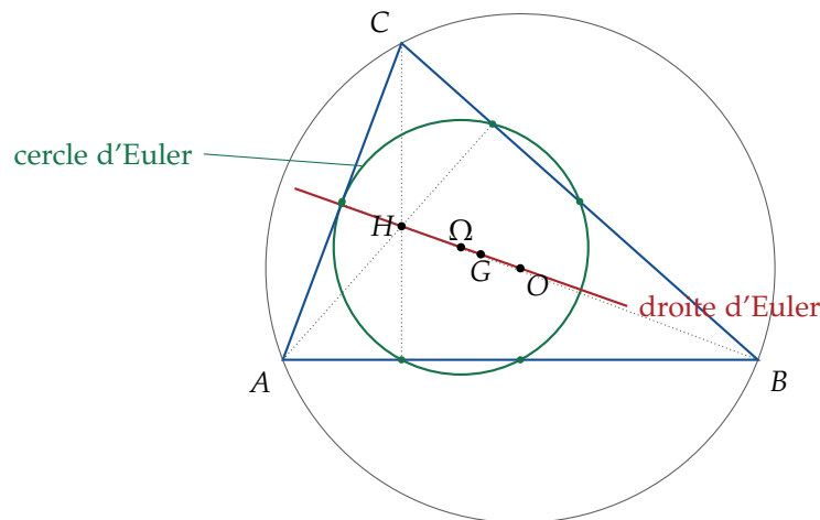
Figure 5.2. Droite d'Euler ( OGH ), avec \overrightarrow{OH} = 3\overrightarrow{OG} , et cercle des neuf points (vert), de centre \Omega milieu de [OH] et de rayon R/2 ; il passe par les milieux des côtés et les pieds des hauteurs (points verts).
