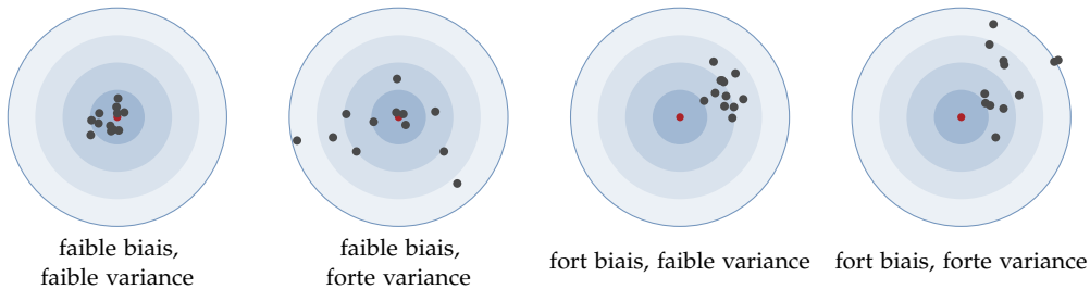
Figure 1.1. Biais et variance comme précision d'un tir : le centre rouge est g(\theta) , chaque point une réalisation de \hat{g} sur un échantillon différent. Le biais est le décalage du nuage, la variance sa dispersion ; le risque quadratique mesure l'écart moyen au centre et additionne les deux (proposition 1.4).
