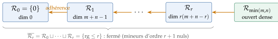
Figure 4.2. Stratification de \mathcal{M}_{m,n}(\mathbb{K}) par le rang ( \mathbb{K} = \mathbb{R} ou \mathbb{C} ) : les orbites de l'action par équivalence sont les \mathcal{R}_r , et l'adhérence d'une orbite est la réunion des orbites de rang inférieur. Chaque flèche se lit « s'accumule sur ».
