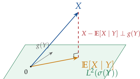
Figure 4.1. L'espérance conditionnelle comme projection orthogonale de X sur le sous-espace des variables de carré intégrable fonctions de Y : l'erreur de prédiction est orthogonale à toute fonction de Y .
