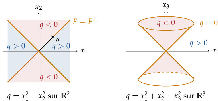
Figure 1.1. Cônes isotropes. À gauche, deux droites ; la droite F = \text{Vect}(1, 1) est son propre orthogonal. À droite, un cône de révolution (le « cône de lumière ») séparant les régions q > 0 et q < 0 .
