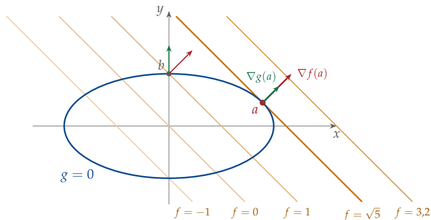
Figure 4.3. Maximiser f(x, y) = x + y sur l'ellipse g(x, y) = \frac{x^2}{4} + y^2 - 1 = 0 . Au point b , la ligne de niveau de f traverse la contrainte : en se déplaçant sur l'ellipse on fait croître ou décroître f , ce n'est pas un extremum. Au maximum a , la ligne de niveau f = \sqrt{5} est tangente à l'ellipse : \nabla f(a) et \nabla g(a) sont colinéaires.
