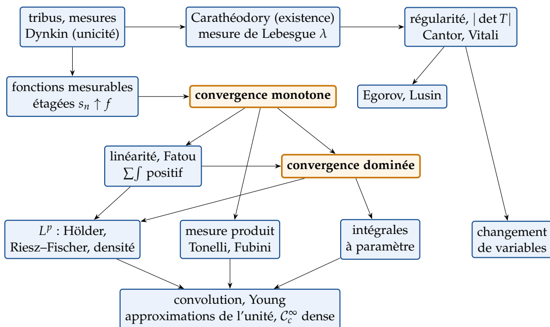
Figure 8.1. L'arbre des dépendances du cours. Les deux théorèmes encadrés en orange portent tout l'édifice.
