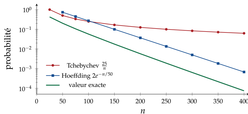
Figure 3.1. \mathbb{P}(|\bar{X}_n - \frac{1}{2}| \geq 0,1) pour n lancers d'une pièce équilibrée, en échelle logarithmique : la borne de Tchebychev décroît en \frac{1}{n} , celle de Hoeffding exponentiellement, comme la vraie valeur (calculée exactement).
