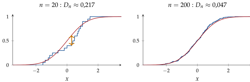
Figure 7.1. Fonction de répartition empirique \mathbb{F}_n (en escalier, bleu) d'échantillons \mathcal{N}(0,1) simulés et fonction de répartition théorique \Phi (rouge). La flèche orange montre l'écart maximal D_n = \sup |\mathbb{F}_n - \Phi| , atteint juste avant un saut. Glivenko–Cantelli : D_n \rightarrow 0 p.s.; Kolmogorov : D_n est de l'ordre de 1/\sqrt{n} .
