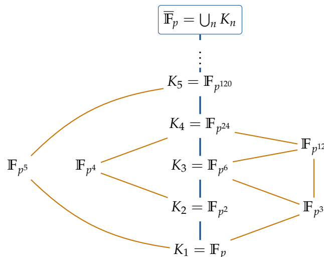
Figure 2.3. La clôture algébrique de \mathbb{F}_p comme réunion. En bleu, la tour K_n = \mathbb{F}_{p^{n!}} de la construction ; en orange, quelques autres corps finis, chacun inclus dans un K_n dès que son degré divise n! . Tous les corps finis de caractéristique p vivent ensemble dans \overline{\mathbb{F}}_p , ordonnés par la divisibilité des degrés.
