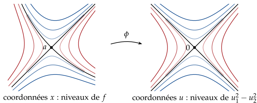
Figure 5.3. Lemme de Morse en dimension 2, indice 1. À gauche, les lignes de niveau de f près d'un point selle non dégénéré : des « hyperboles déformées ». Le difféomorphisme \phi les redresse en les hyperboles exactes u_1^2 - u_2^2 = c ; en particulier le niveau critique est formé de deux courbes régulières se coupant transversalement en a .
