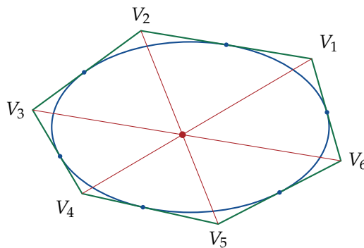
Figure 5.4. Théorème de Brianchon, dual de Pascal : les diagonales d'un hexagone circonscrit à une conique sont concourantes.
