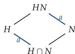
Figure 2.3. Le deuxième théorème d'isomorphisme, ou « théorème du losange ».
