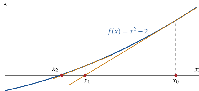
Figure 13.1. Méthode de Newton pour x^2 = 2 (méthode de Héron) : on remplace la courbe par sa tangente. x_0 = 2,5 , x_1 = 1,65 , x_2 \approx 1,4311 , x_3 \approx 1,41421 : le nombre de décimales exactes double à chaque pas. Ici f est convexe croissante et x_0 \geq \sqrt{2} : la convergence est globale et monotone.
