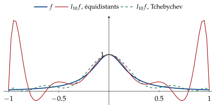
Figure 6.1. Phénomène de Runge pour f(x) = \frac{1}{1+25x^2} , n = 10 : avec des nœuds équidistants, l'erreur uniforme vaut 1,92 (oscillations au bord); avec les nœuds de Tchebychev, 0,11.
