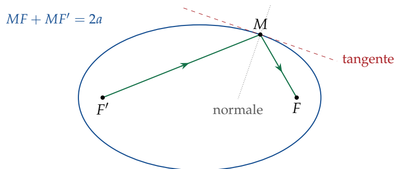
Figure 7.2. Propriété bifocale et propriété optique : la normale en M est la bissectrice intérieure de \widehat{FMF'} , donc un rayon issu de F' se réfléchit en passant par F .
