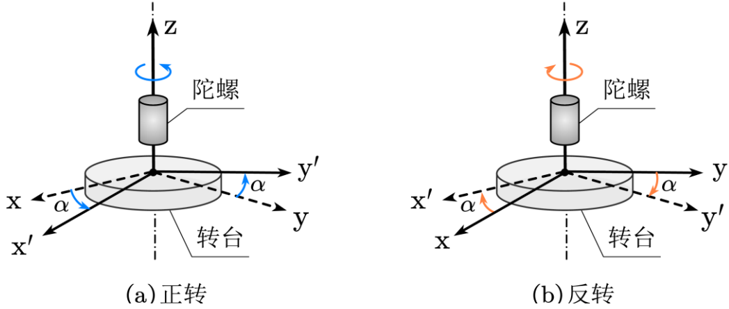
图 3 z 轴陀螺敏感轴朝上，转台分别绕 z 轴正方向转动 \alpha 角和绕 z 轴正方向反转 \alpha 角
