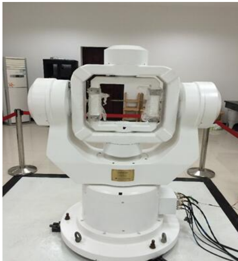
图 1 高精度三轴转台
