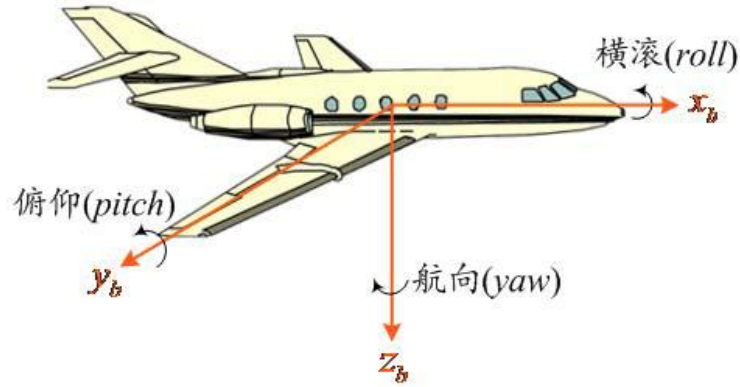
图 4 载体的坐标轴及姿态角示意图（假设 IMU 的 x , y , z 轴分别与飞机载体 x , y , z 轴对齐）
