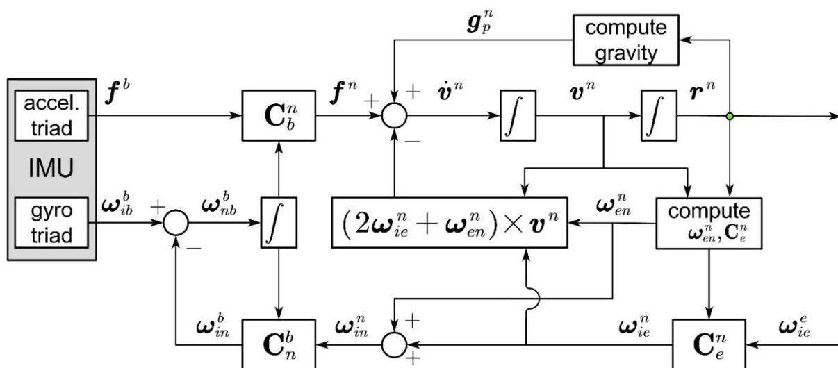
图 5 纯惯导算法原理图
