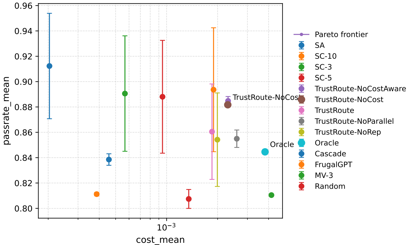
GSM8K
