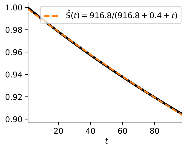
Human, PacBio HiFi
