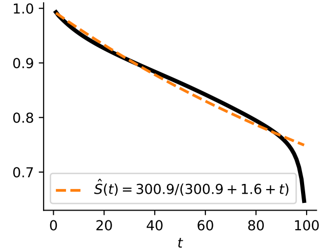
B. subtilis , Illumina
