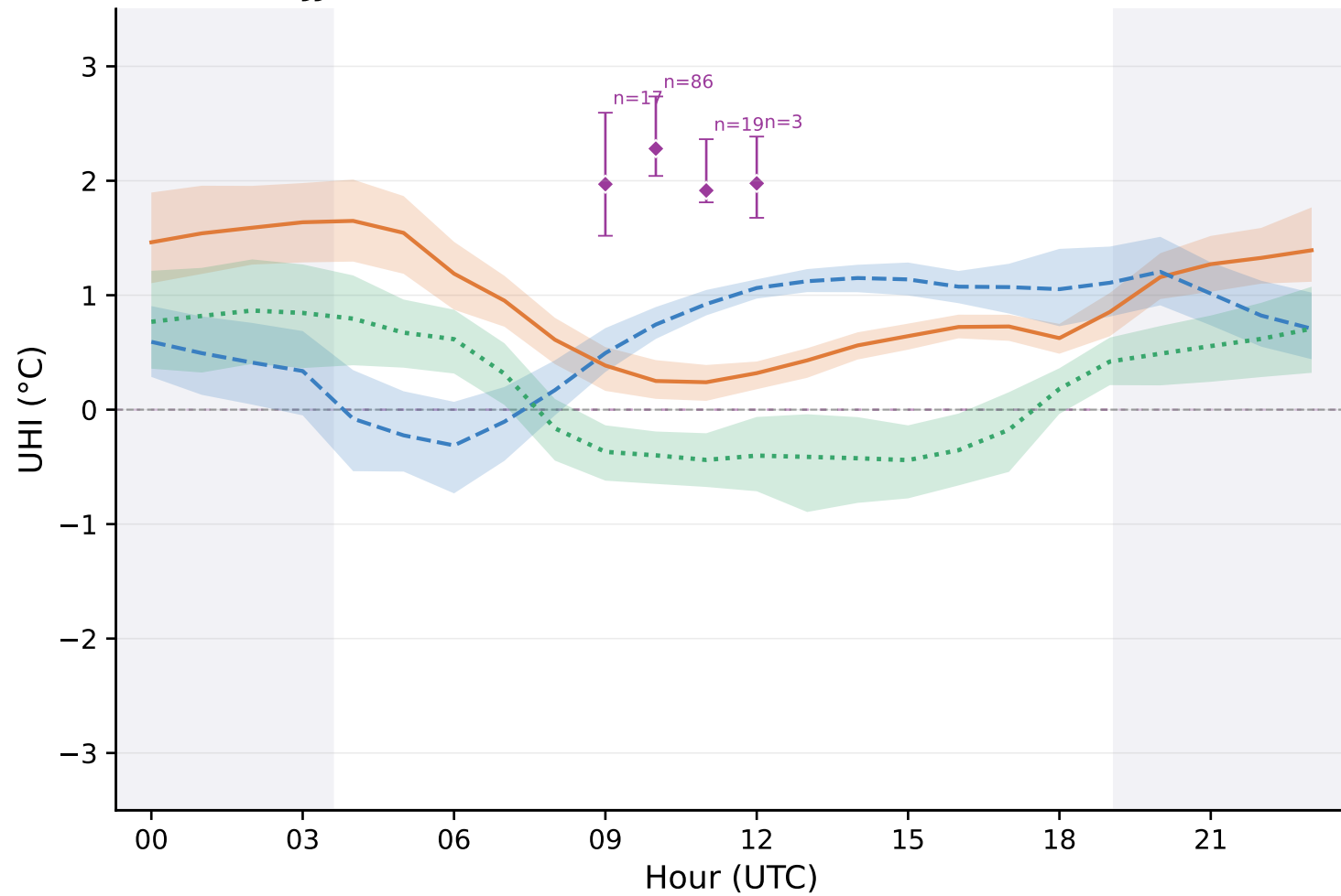
Summer (JJA)
