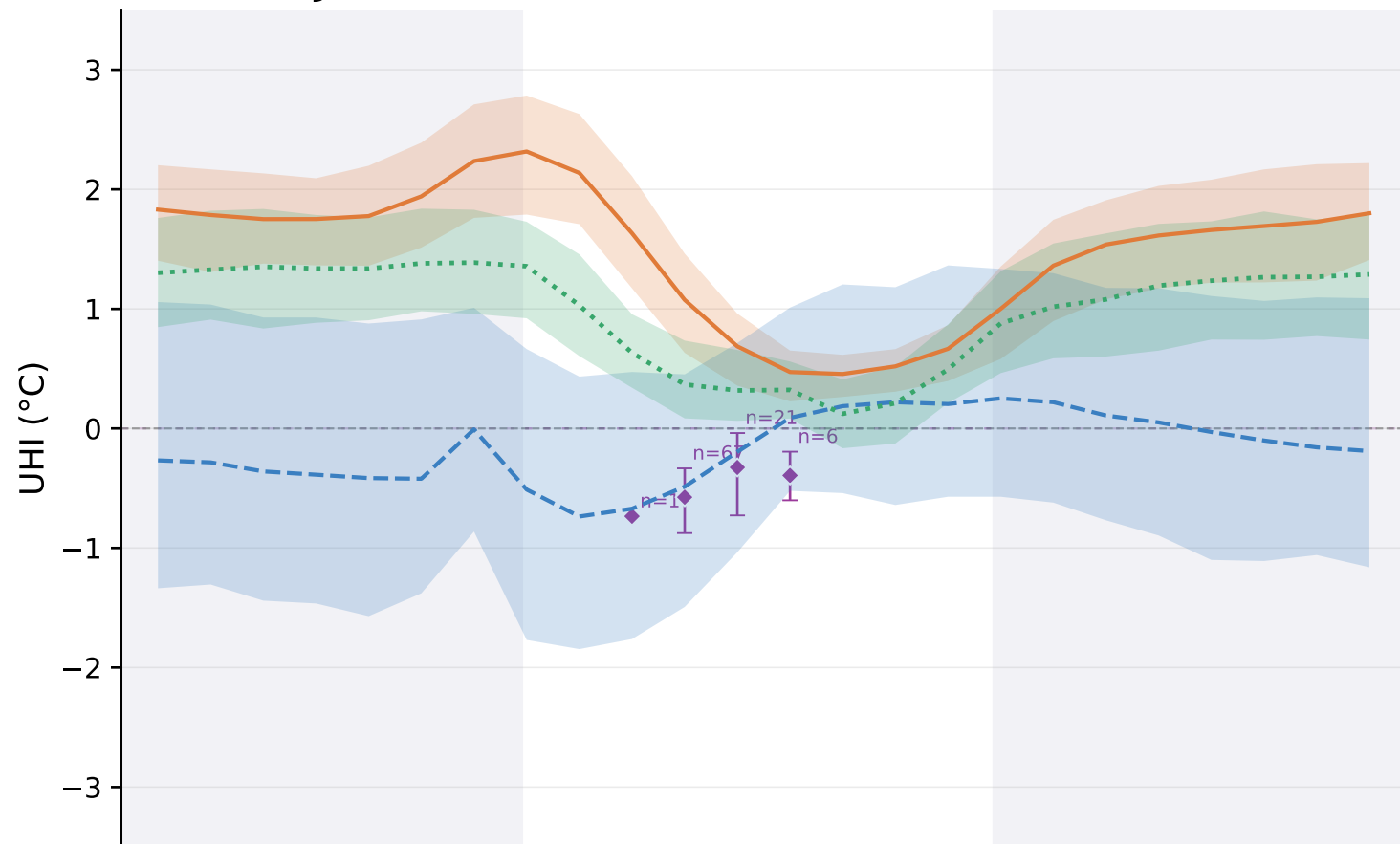
Winter (DJF)
