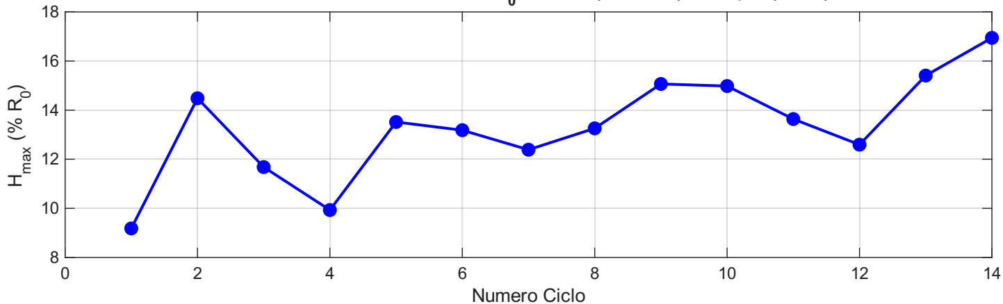
Errore Massimo di Isteresi su R_0 Globale (9439.5 \Omega ) - 12 cpm (corto)
