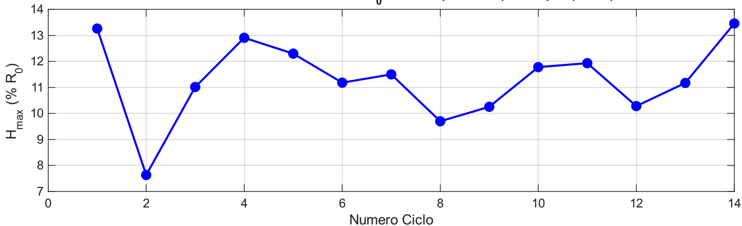
Errore Massimo di Isteresi su R_0 Globale (9439.5 \Omega ) - 24 cpm (corto)
