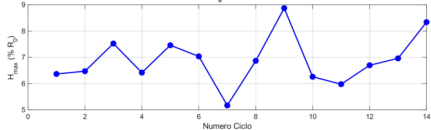
Errore Massimo di Isteresi su R_0 Globale (9439.5 \Omega ) - 48 cpm (corto)
