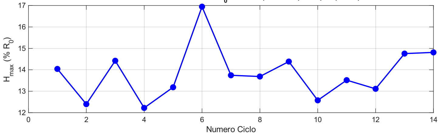
Errore Massimo di Isteresi su R_0 Globale (9439.5 \Omega ) - 6 cpm (corto)
