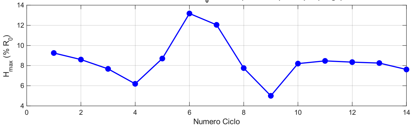
Errore Massimo di Isteresi su R_0 Globale (19072.1 \Omega ) - 24 cpm (lungo)
