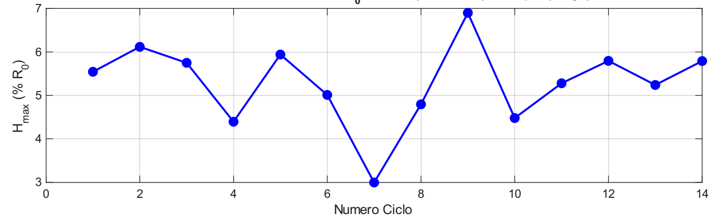
Errore Massimo di Isteresi su R_0 Globale (19072.1 \Omega ) - 60 cpm (lungo)
