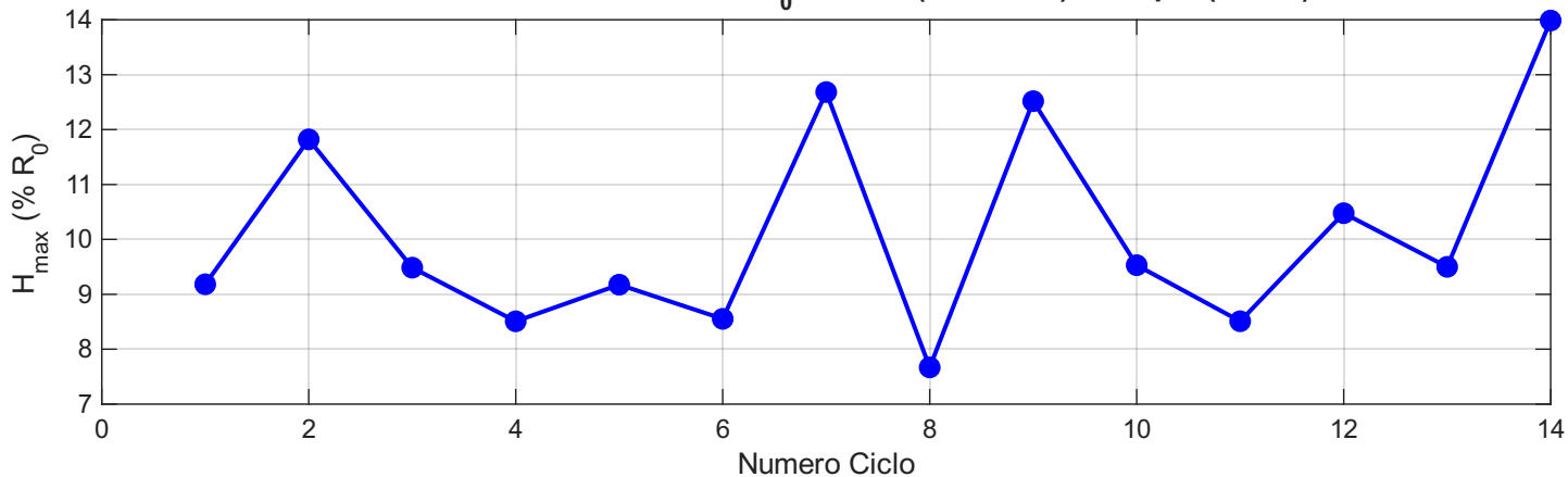
Errore Massimo di Isteresi su R_0 Globale (13240.6 \Omega ) - 12 cpm (medio)
