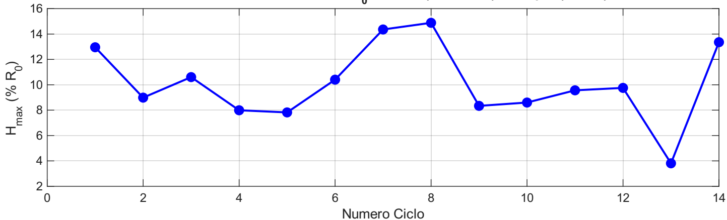
Errore Massimo di Isteresi su R_0 Globale (13240.6 \Omega ) - 24 cpm (medio)
