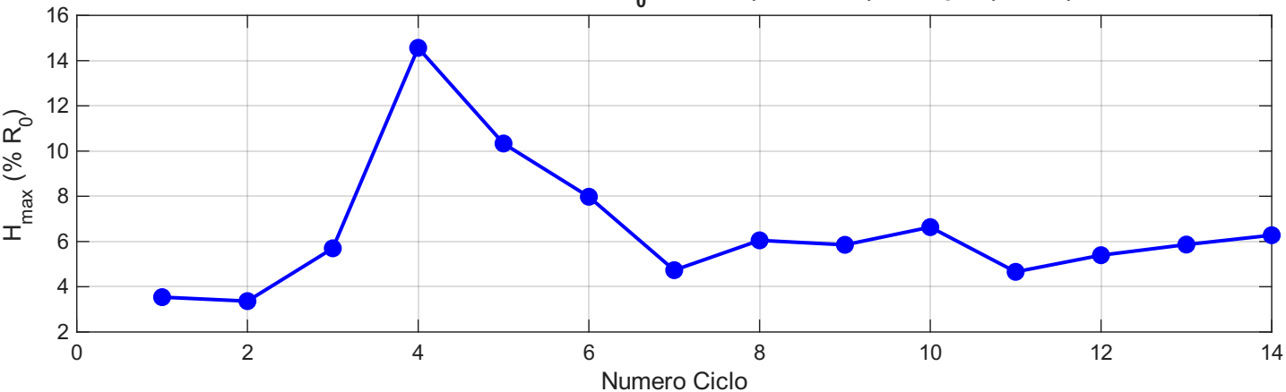
Errore Massimo di Isteresi su R_0 Globale ( 13240.6 \Omega ) - 48 cpm (medio)
