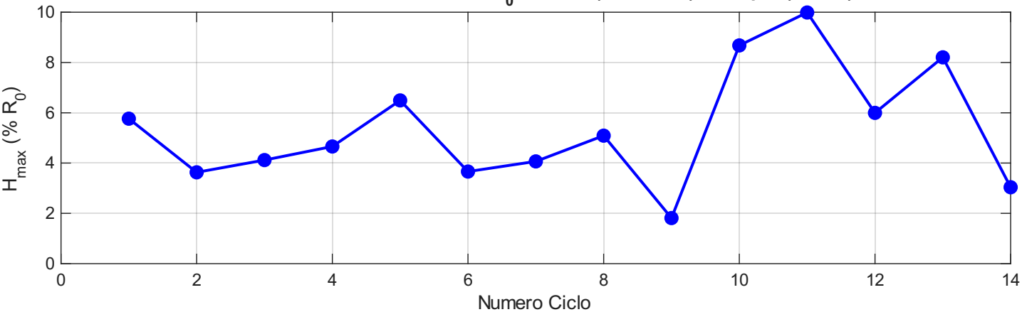
Errore Massimo di Isteresi su R_0 Globale (13240.6 \Omega ) - 60 cpm (medio)
