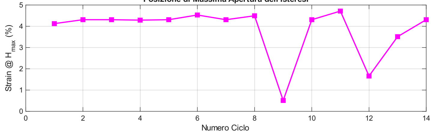
Posizione di Massima Apertura dell'Isteresi
