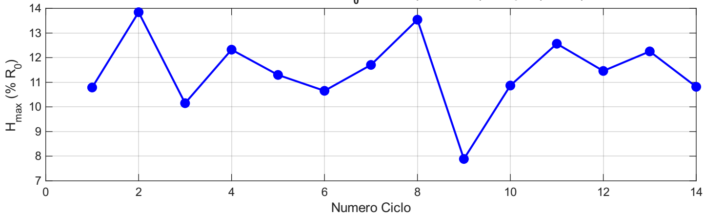
Errore Massimo di Isteresi su R_0 Globale ( 13240.6 \Omega ) - 6 cpm (medio)
