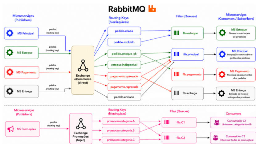
Figura 2 – Comunicação indireta entre os processos
