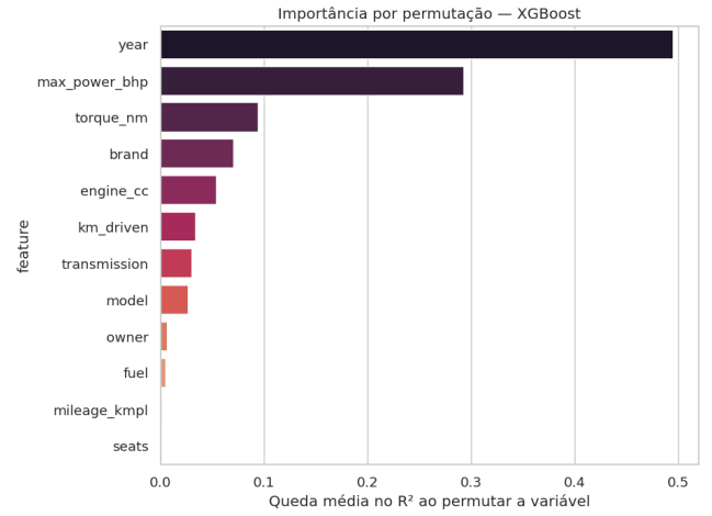
Fig. 5. Importância por permutação das variáveis segundo o melhor modelo (XGBoost): queda média no R^2 ao permutar cada atributo.
