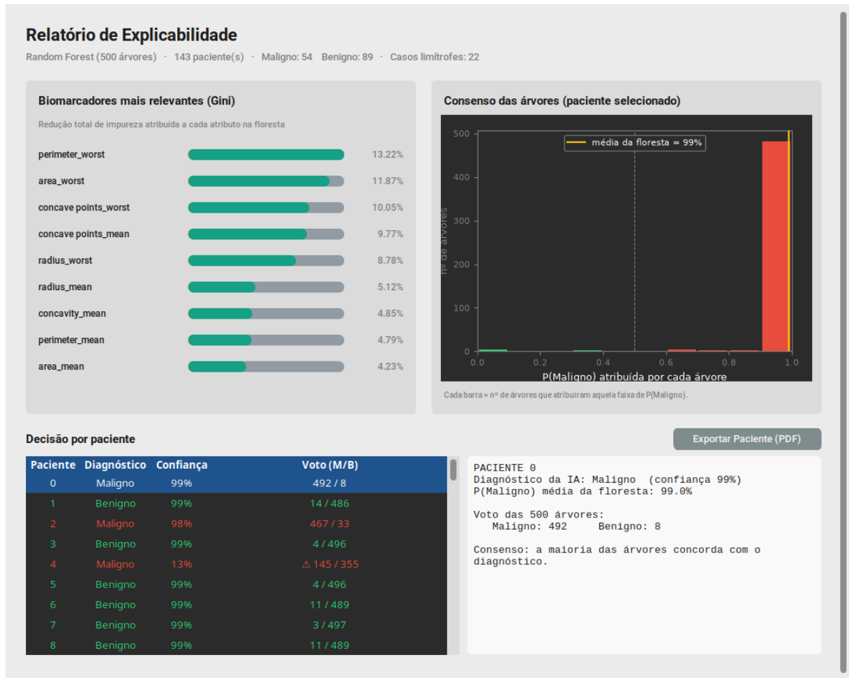
FIGURA 14 – RELATÓRIO DO RANDOM FOREST: CONSENSO ENTRE AS ÁRVORES DA FLORESTA
