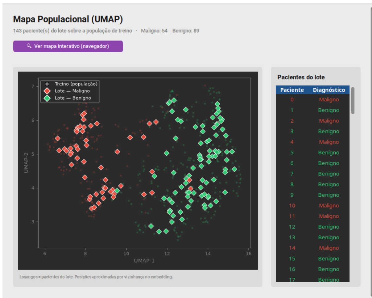
FIGURA 17 – MAPA POPULACIONAL: PROJEÇÃO UMAP DO LOTE SOBRE O CONJUNTO DE TREINO
