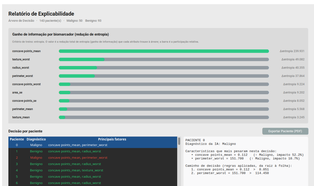
FIGURA 13 – RELATÓRIO DA ÁRVORE DE DECISÃO: GANHO DE INFORMAÇÃO E CAMINHO DE REGRAS
