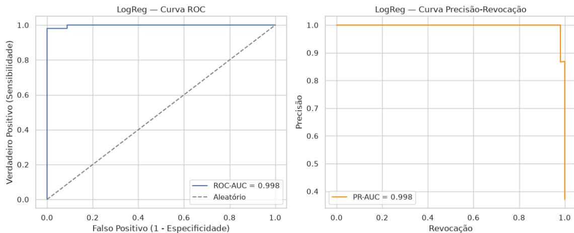
GRÁFICO 4 – CURVAS ROC E PRECISÃO-REVOCAÇÃO DA REGRESSÃO LOGÍSTICA
