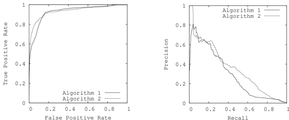
FIGURA 4 – COMPARAÇÃO ENTRE CURVAS ROC E PRECISÃO-REVOCAÇÃO EM DADOS DESBALANCEADOS
