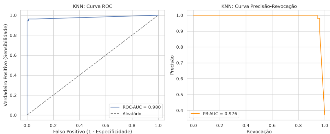
GRÁFICO 3 – CURVAS ROC E PRECISÃO-REVOCAÇÃO DO KNN
