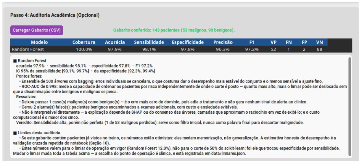
FIGURA 18 – AUDITORIA ACADÊMICA: DESEMPENHO DOS MODELOS CONTRA O GABARITO
