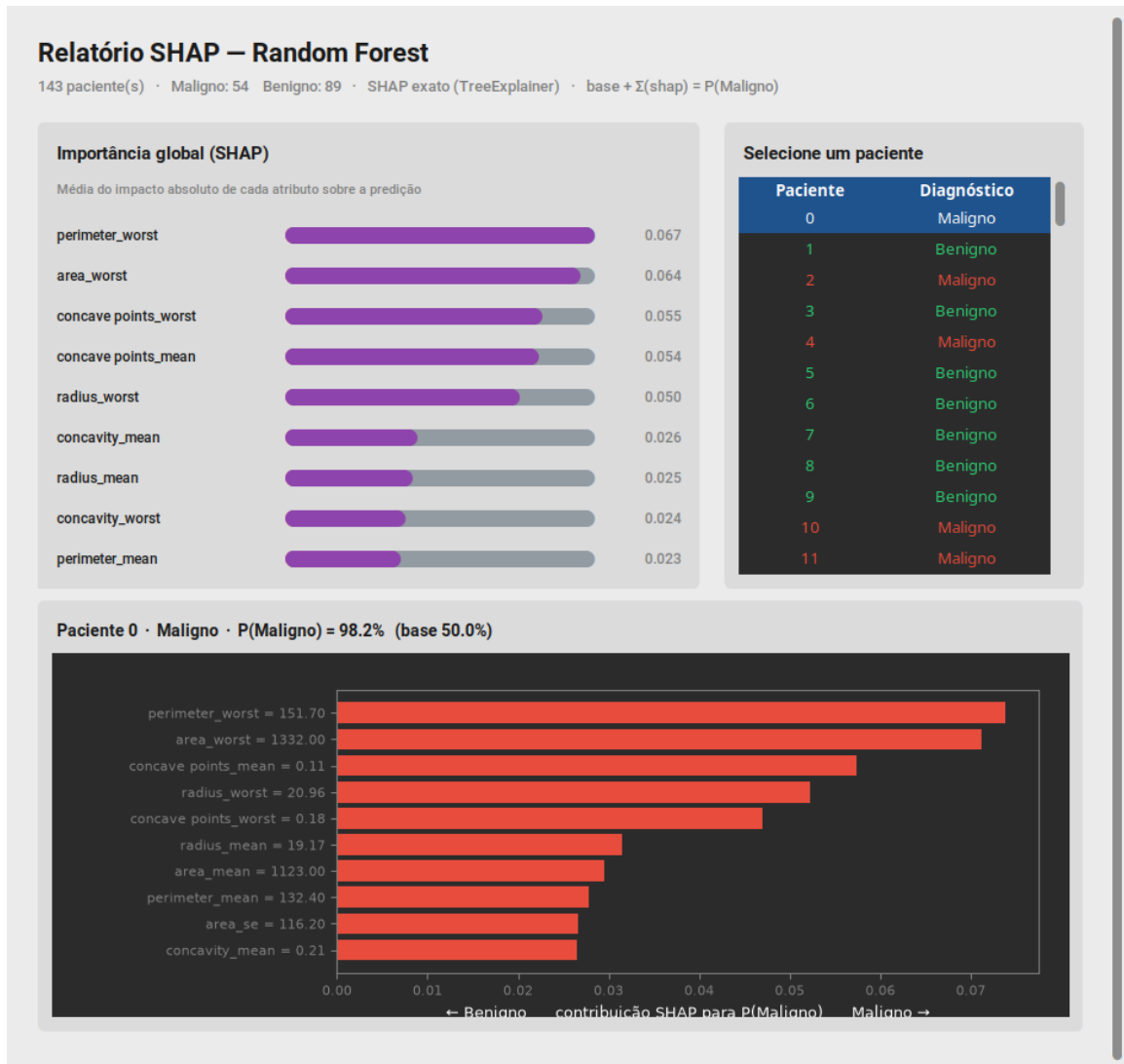
FIGURA 16 – RELATÓRIO SHAP: IMPORTÂNCIA GLOBAL E CONTRIBUIÇÃO POR PACIENTE
