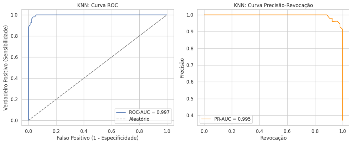
FIGURA 13 – CURVAS ROC E PRECISÃO-REVOCAÇÃO DO KNN
