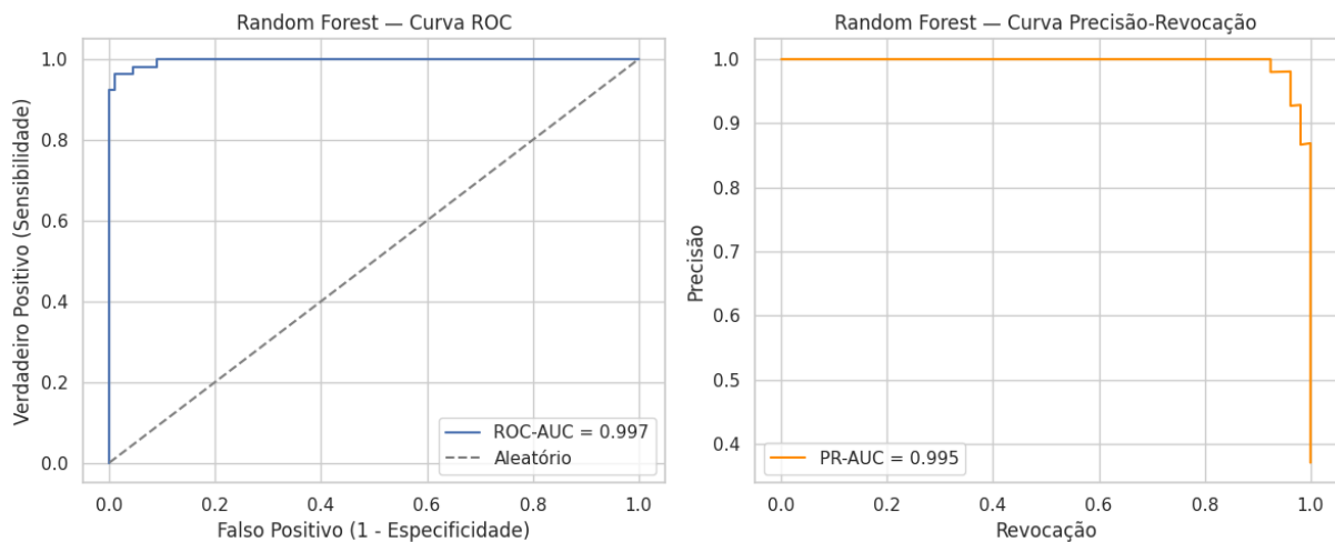
FIGURA 15 – CURVAS ROC E PRECISÃO-REVOCAÇÃO DO RANDOM FOREST
