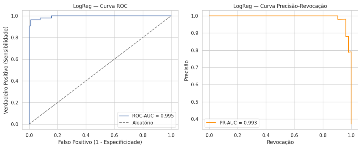
FIGURA 14 – CURVAS ROC E PRECISÃO-REVOCAÇÃO DA REGRESSÃO LOGÍSTICA
