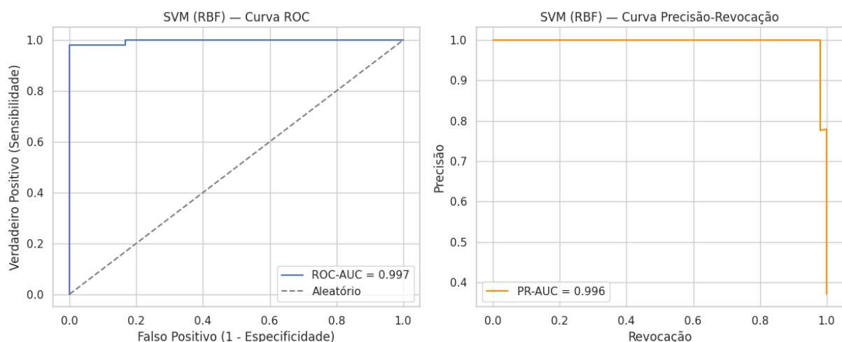
FIGURA 16 – CURVAS ROC E PRECISÃO-REVOCAÇÃO DO SVM
