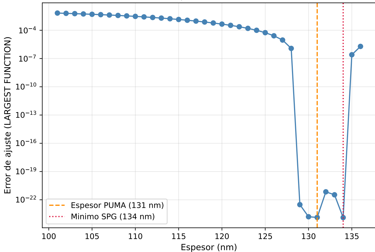
Barrido de espesor en \lambda=550 nm — S5
