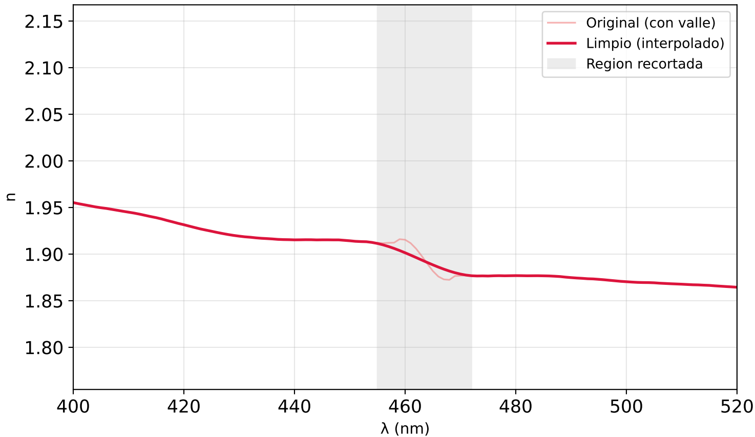
Limpieza manual del valle en n(\lambda)
