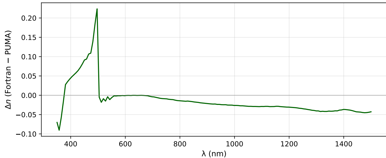
Diferencia Fortran - PUMA (malla comun, 150 puntos) — S2 — 10 sccm O 2
