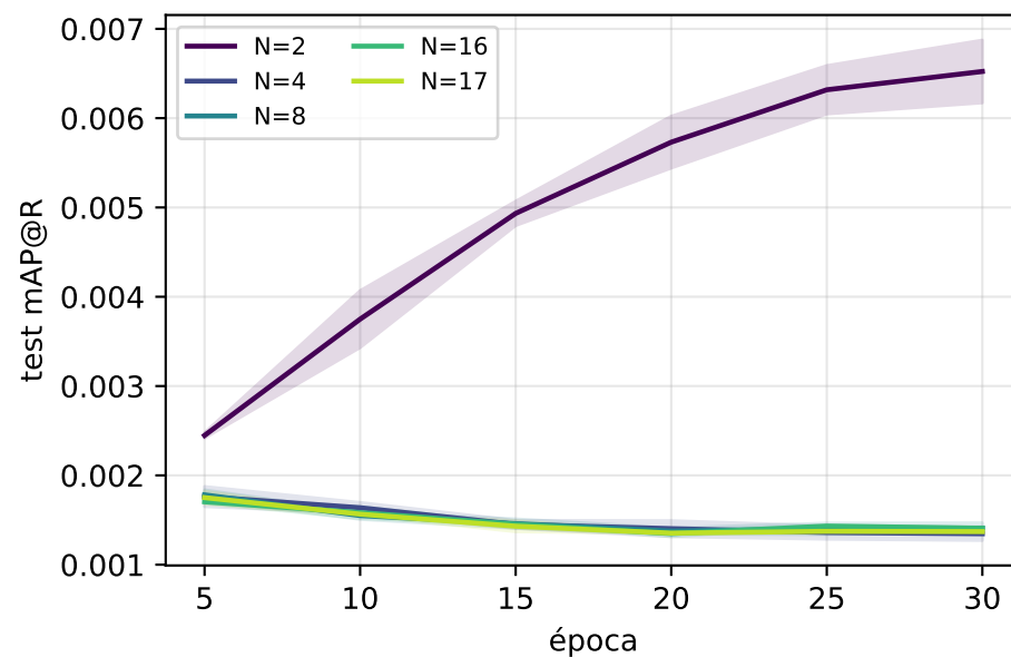
cub200 · mds
