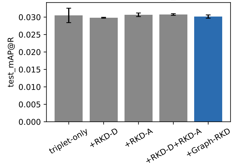
cub200 · convnext_tiny
