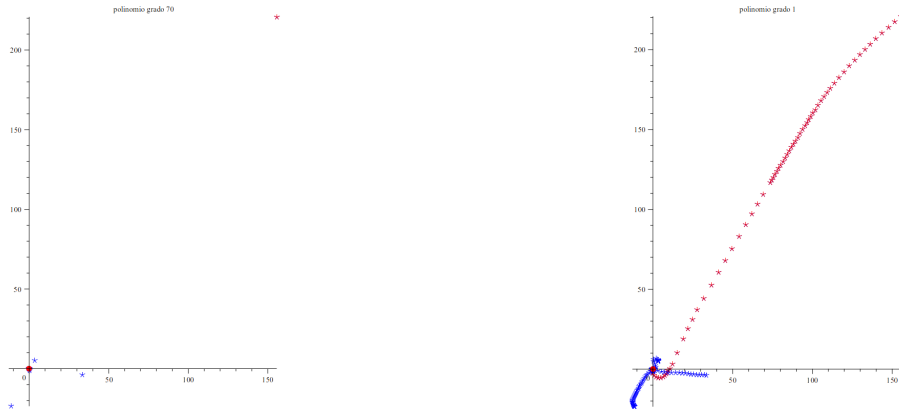
(a) Conjunto de ceros de \varphi_{70} .
