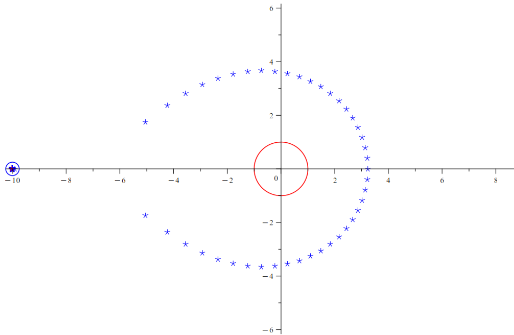
polinomio grado 70
